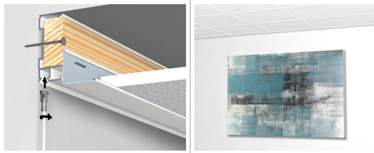
ART STRIP (ICM SYSTEEMPLAFOND)
